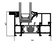
Okno otvíravé – řez
