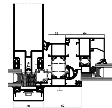
Okno ve fasádě – řez
